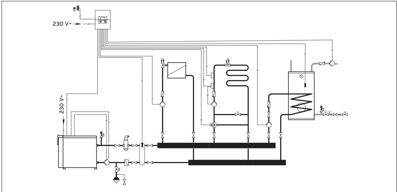
Hidrolik karıştırıcıli hidrolik şeması
