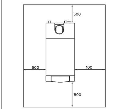
Kurulum sırasında önerilen mesafeler (mm olarak)
