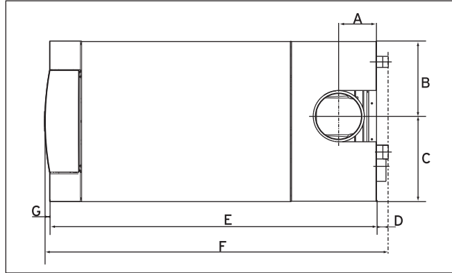
Cihaz ölçüsü
