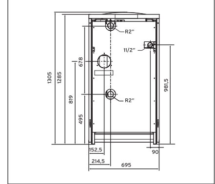
Bağlantı ölçüsü (mm olarak)
